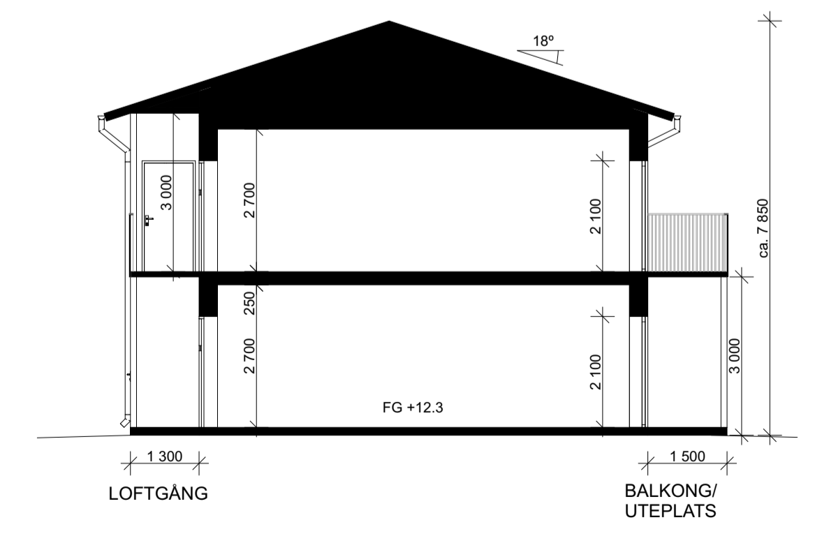
SEKTION B-B
