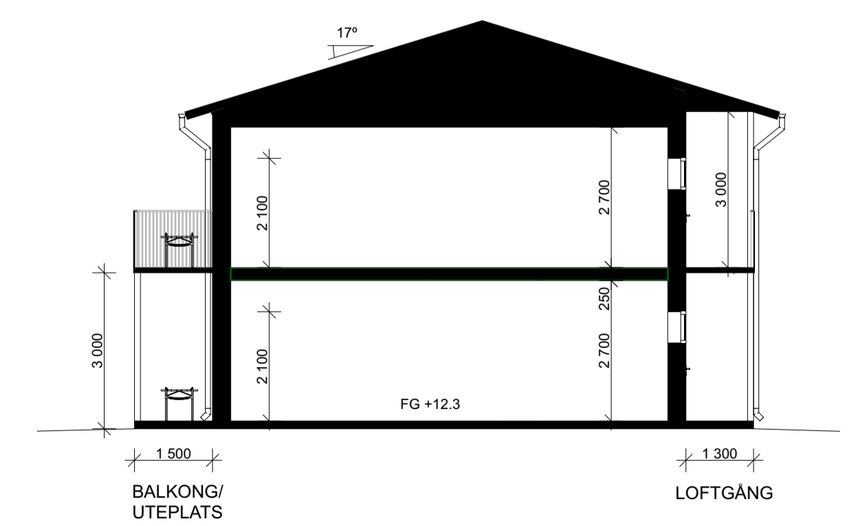
SEKTION A-A
